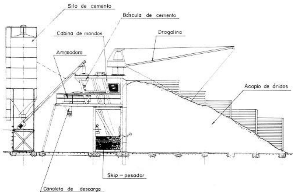
Figura 1. Esquema de una planta hormigonera tipo "radial" con dragalina y amasadora
