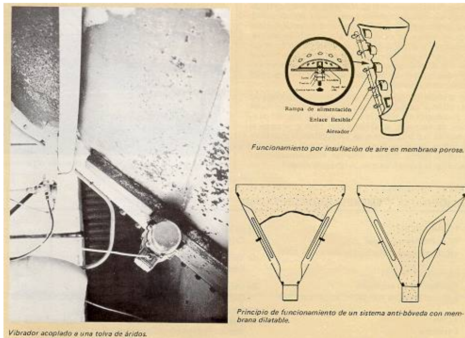
Figura 4. Algunos sistemas anti-bóveda
